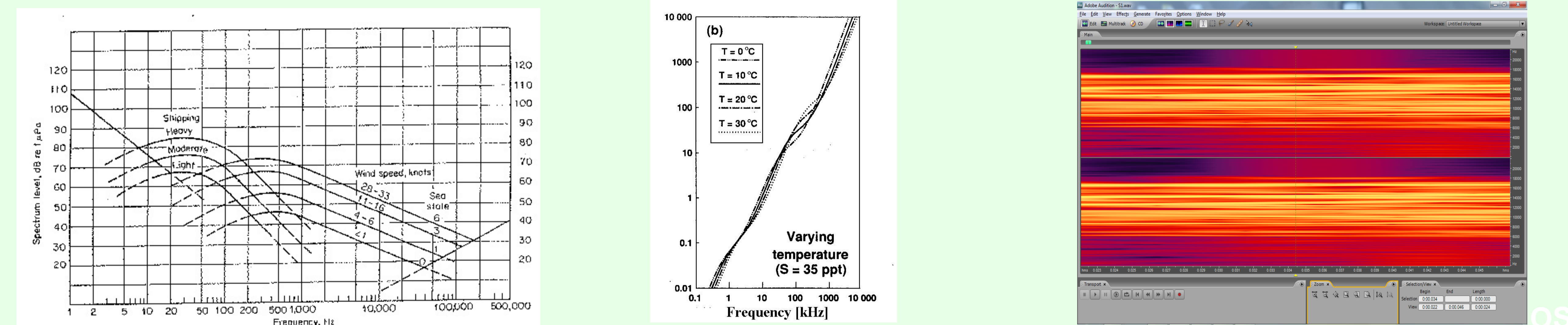
Εικ.2: Μέθοδος υπολογισμού SPL. Στα αριστερά παρουσιάζονται οι καμπύλες Wenz, από τις οποίες υπολογίστηκε ο θόρυβος περιβάλλοντος για την κύρια συχνότητα 12 KHz, αλλά και για την γκάμα συχνοτήτων 0-22000 Hz. Στο κέντρο η γραφική απεικόνιση του συντελεστή απορρόφησης συναρτήσει της θερμοκρασίας. Στα δεξιά παρουσιάζεται κατόπιν μεγένθυσης η κεντρική συχνότητα 12 KHz. Αξίζει να σημειωθεί η «συνέχεια» του ήχου ακόμη και μετά από πολλαπλές μεγενθύνσεις.
